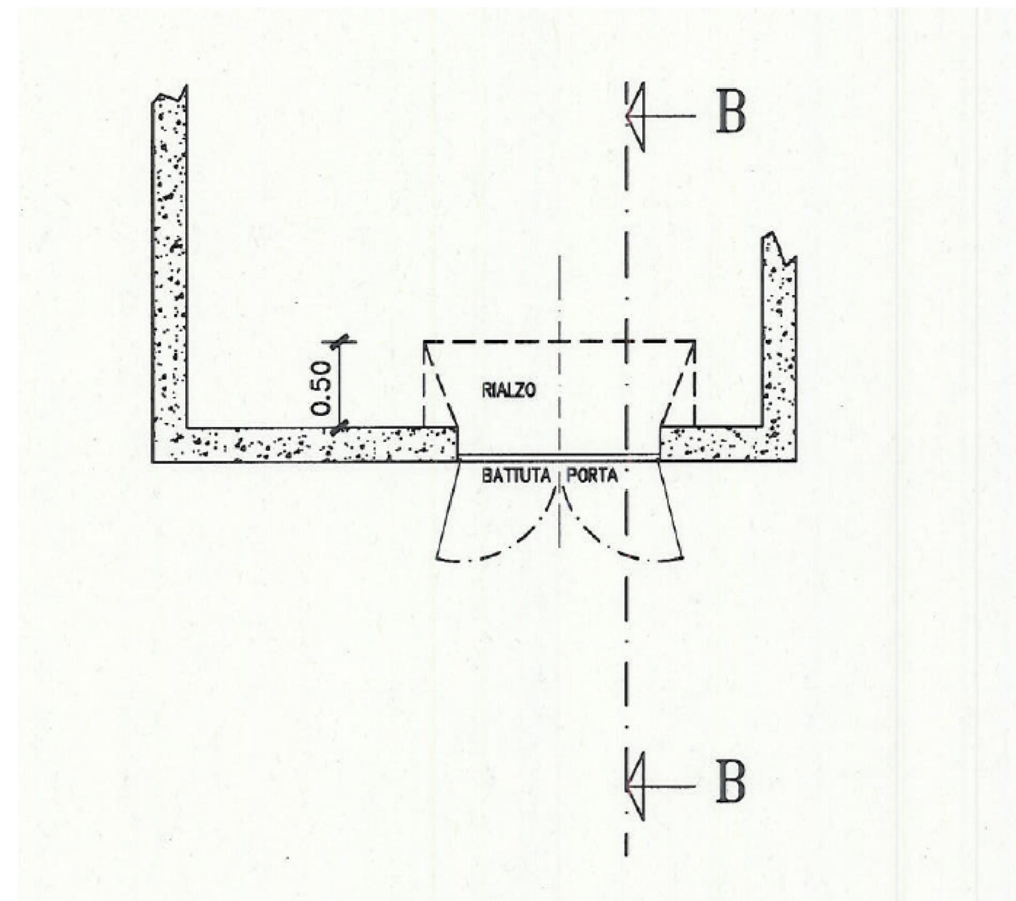
PARTICOLARE SOVRALZO PORTA
