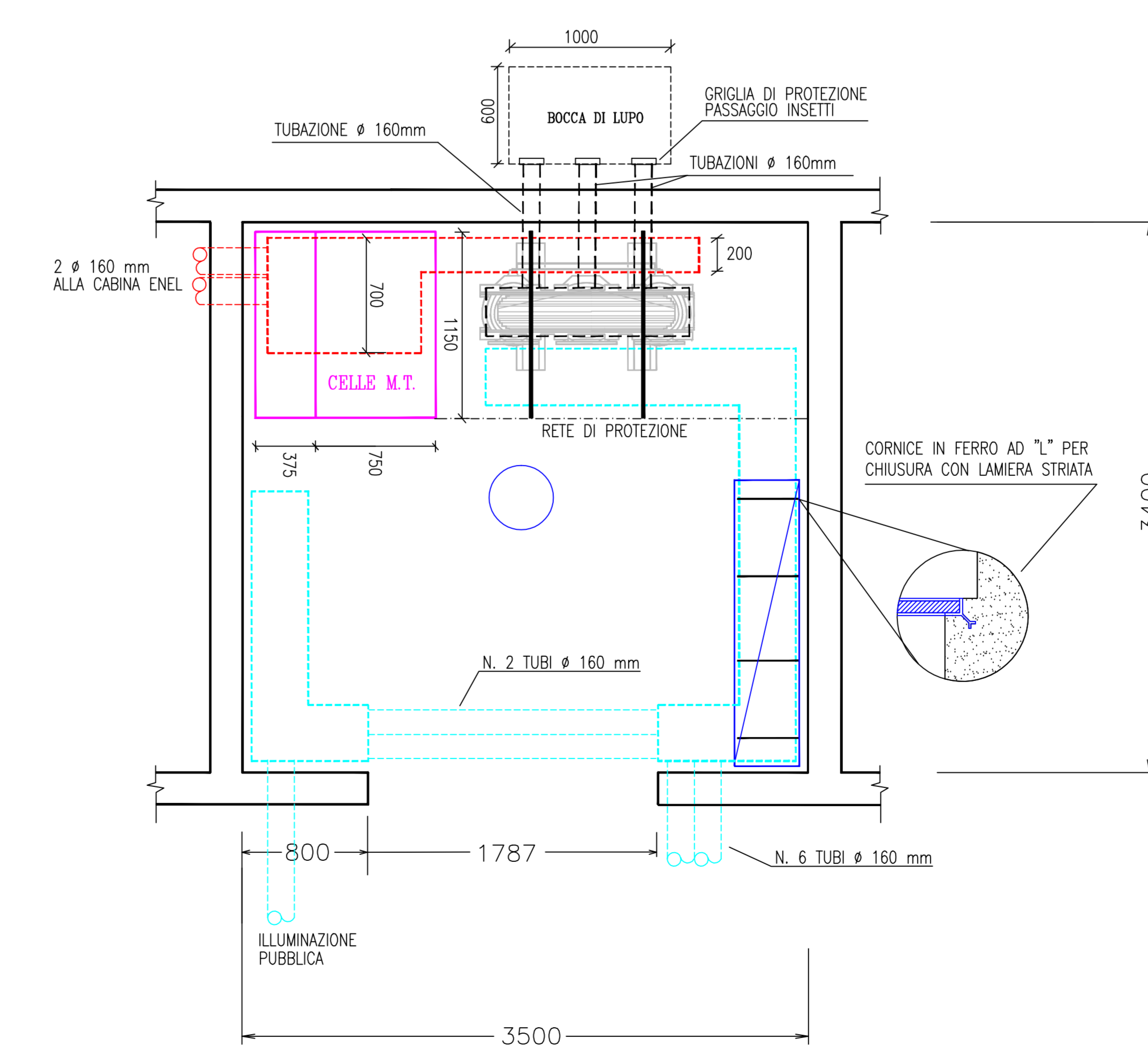
PARTICOLARE INTALLAZIONE IMPIANTI NELLA CABINA DI TRASFORMAZIONE UTENTE
