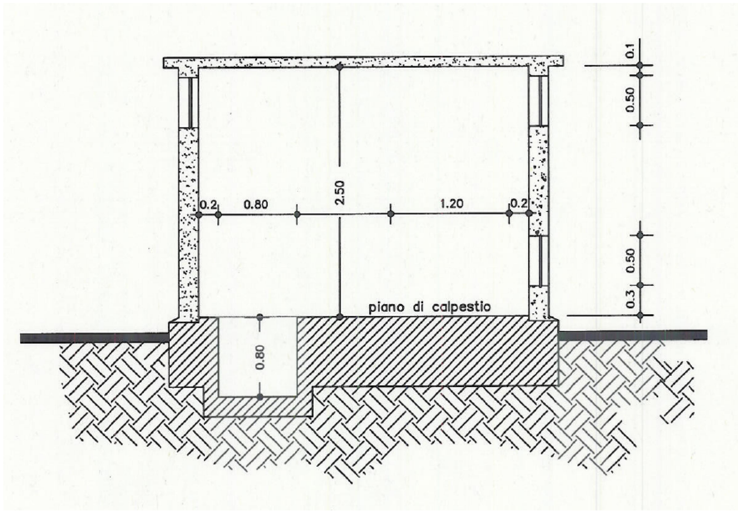
PARTICOLARE SEZIONE A-A
