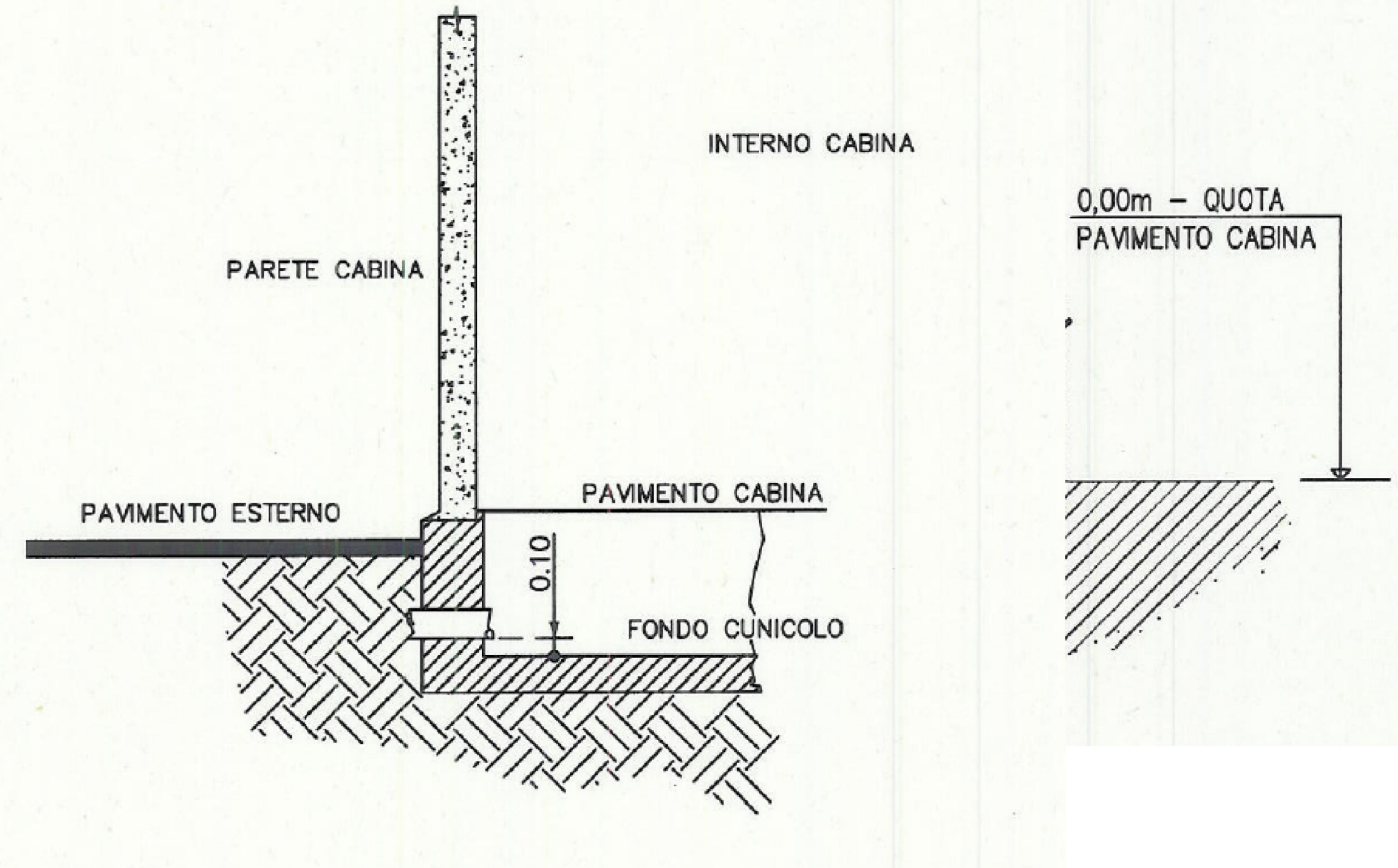
SEZIONE B-B PARTICOLARE SOVRALZO PORTA
