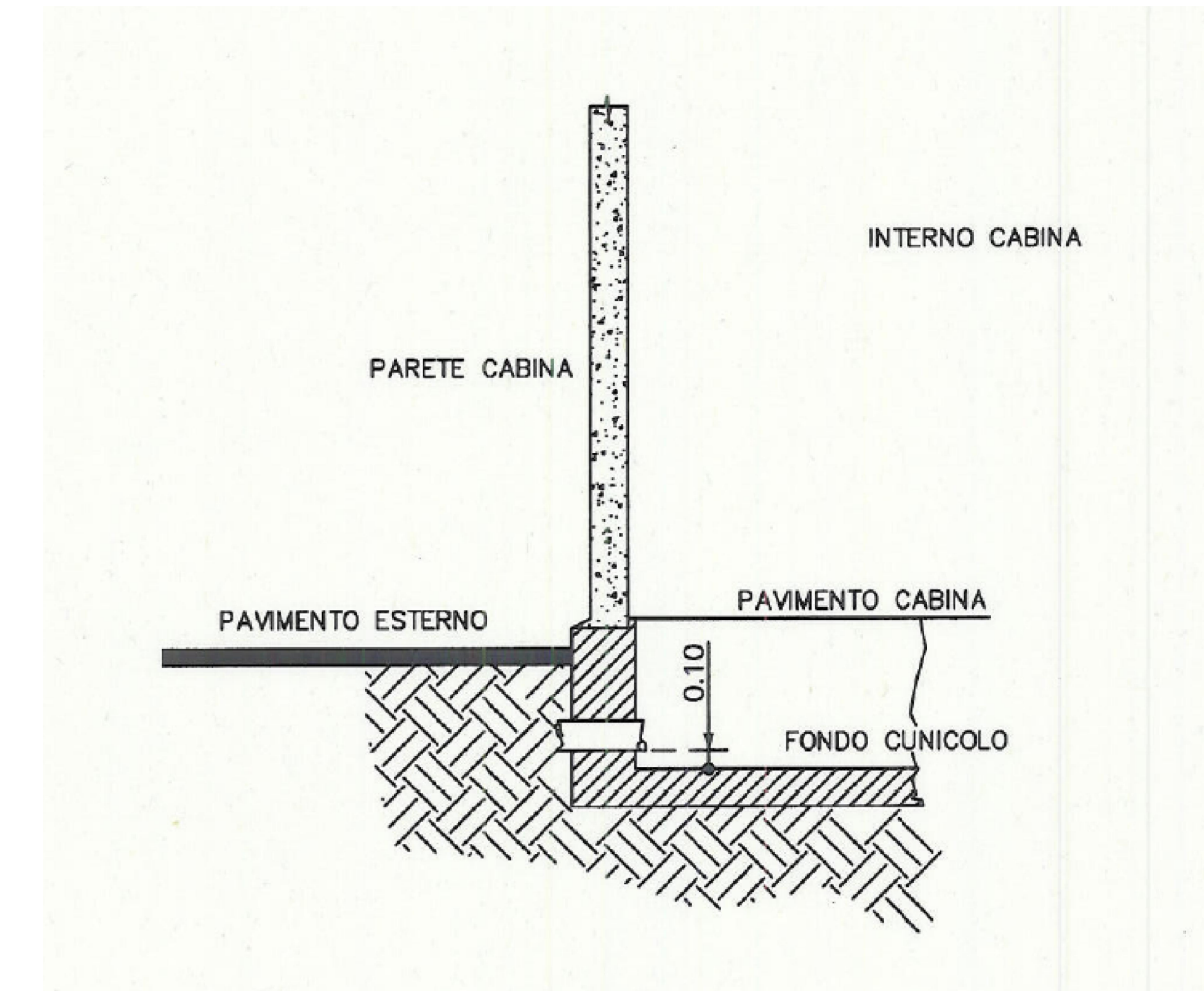
PARTICOLARE INGRESSO TUBI NEL CUNICOLO VISTA IN SEZIONE
