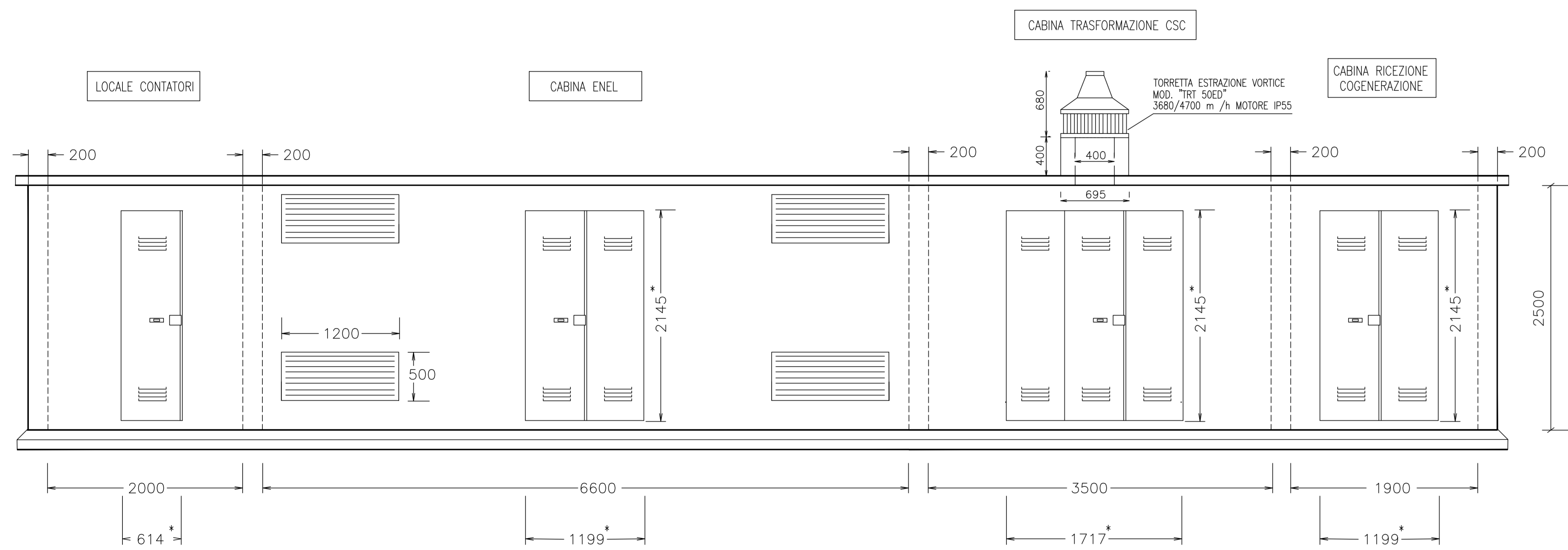
PROSPETTO LATO INGRESSO
