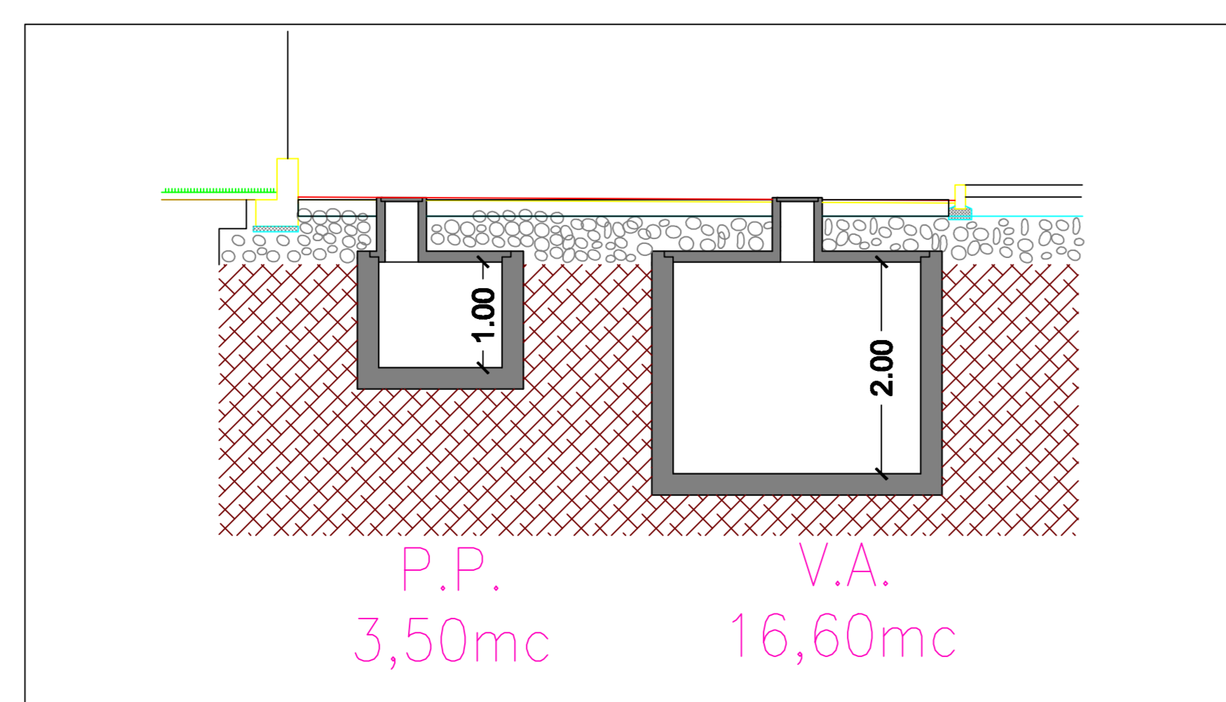
SEZIONE "X-X"
